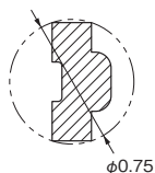
形XC5H ディップ端子断面図
