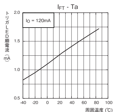
トリガLED順電流－周囲温度
