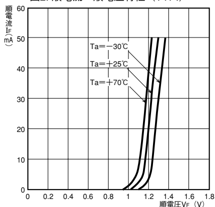
図2. 順電流—順電圧特性 (TYP.)
