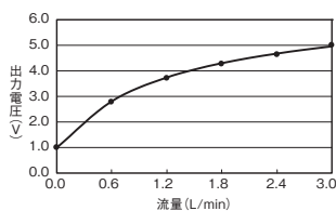
形D6F-03A3-000
