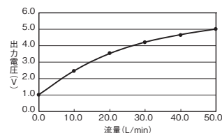
形D6F-05N6-000
