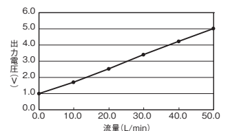
形D6F-05N6-000
