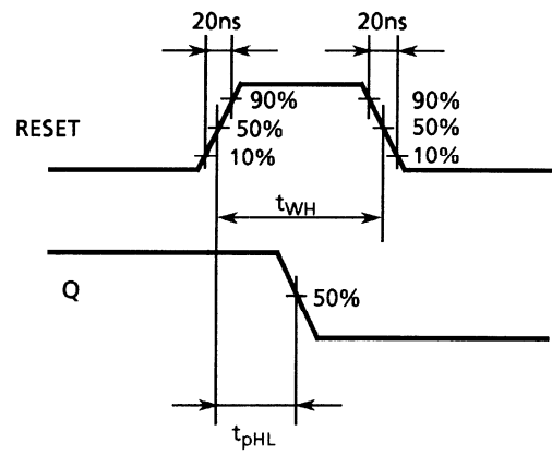
波形 2
