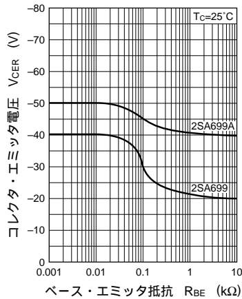
V_{CER} - R_{BE}
