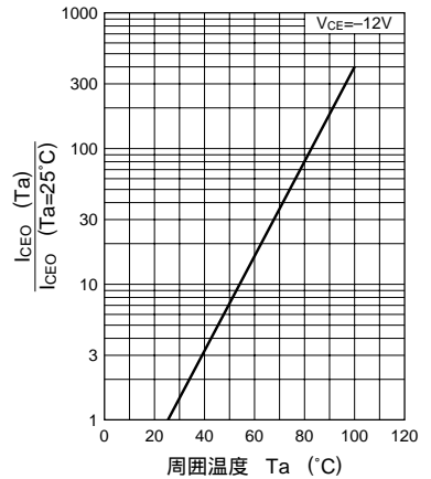
I_{CE0} - T_a
